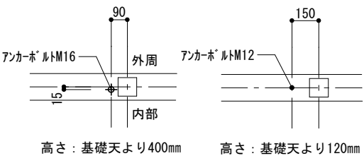
ホルダウン用アンカーボルト配置
